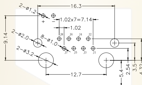
PCB参考图
